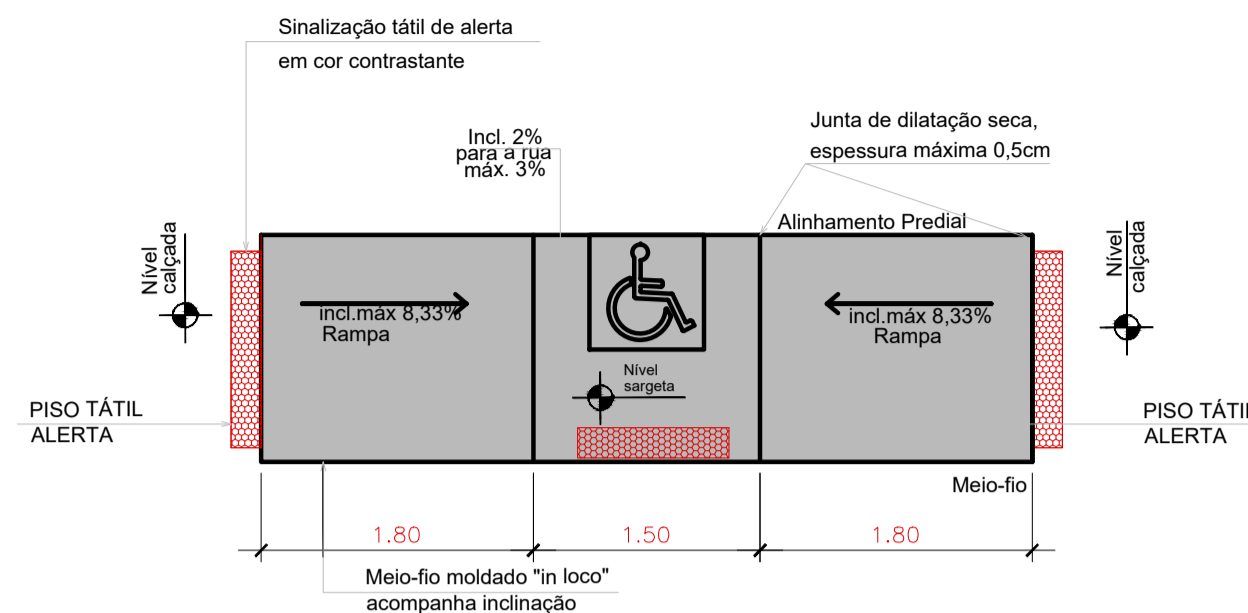
PLANTA BAIXA ESC.1:50
