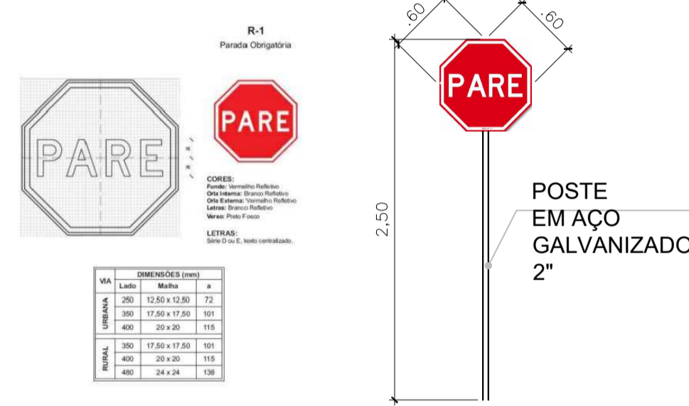
PLACAS- SINALIZAÇÃO VERTICAL 1:50
