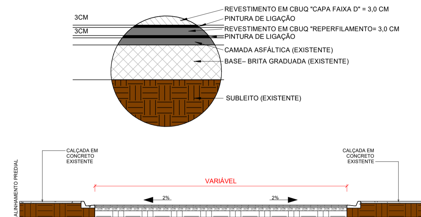
PERFIL RUA RECAPE 1 : 75
