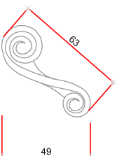
VÓLUTA (V-1) Esc. 1/12,5
