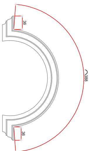
MOLDURA (M-2b) Esc. 1/25
