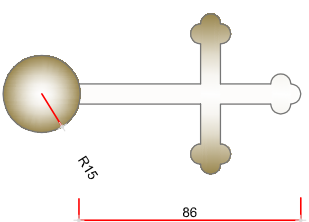
ESFERA (E-2); CRUZ (C-3) Esc. 1/12,5
