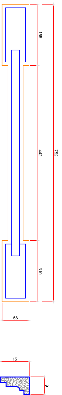
MOLDURA (M-1) Esc. 1/25
