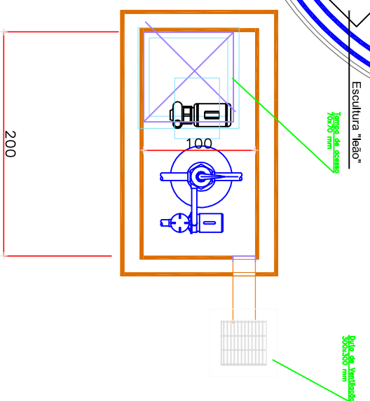
PLANTA DA CASA DE MÁQUINAS Esc. 1/20
