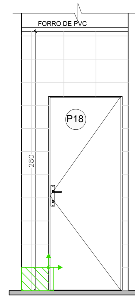
VISTA 03- DML LAVANDERIA "LIMPA" ESC.: 1:25
