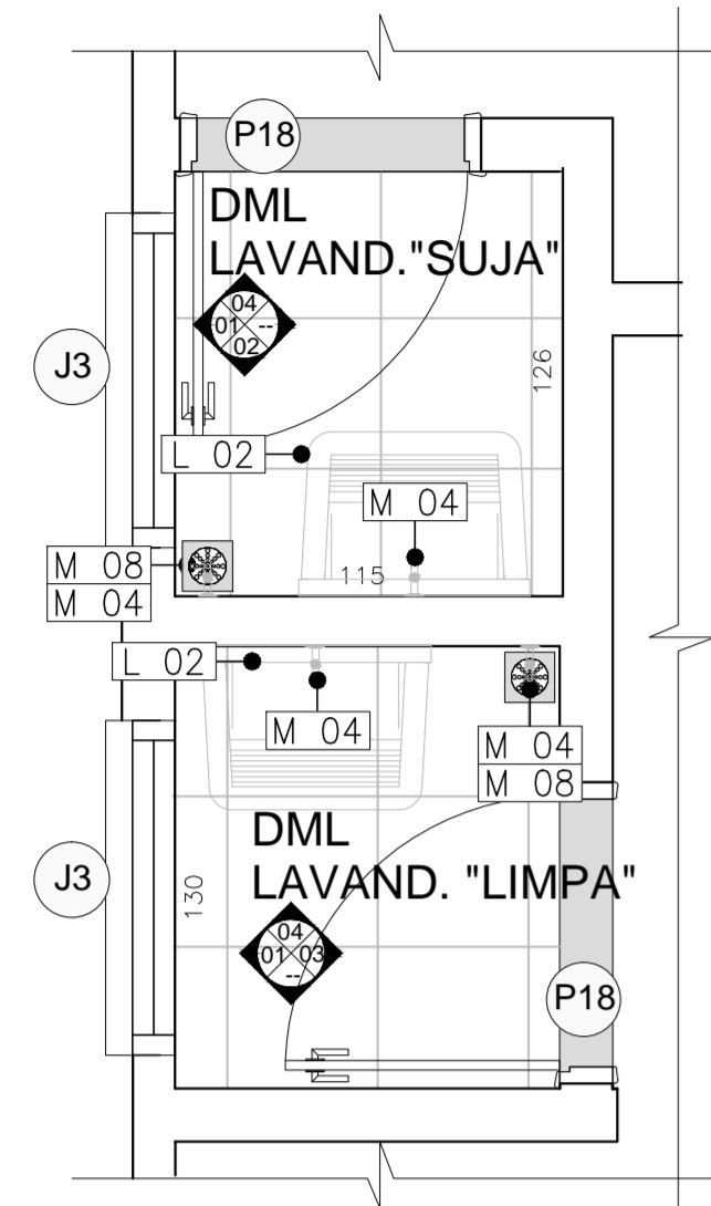
PLANTA BAIXA - DML LAVANDERIA "SUJA" ESC.: 1:25
