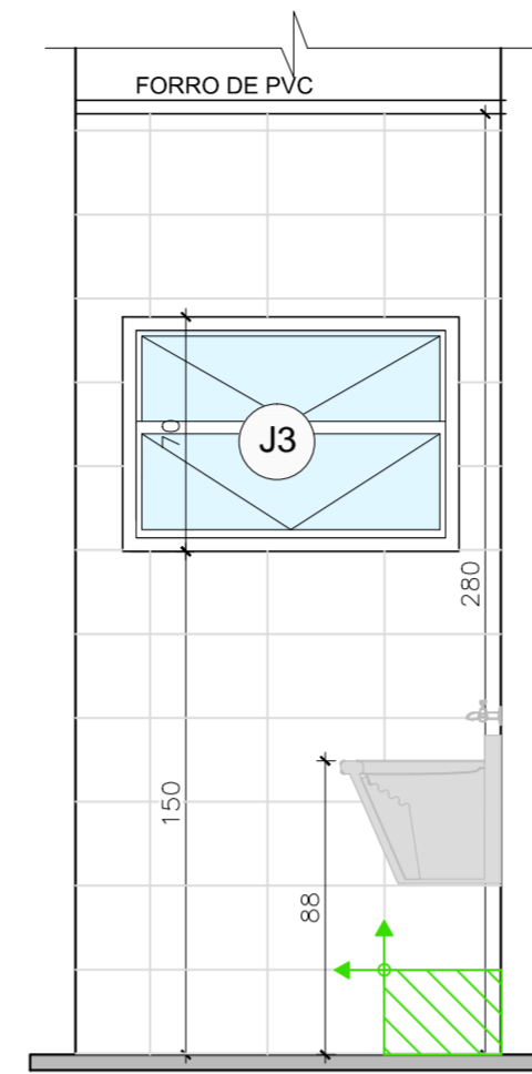
VISTA 01- DML LAVANDERIA "LIMPA" ESC.: 1:25
