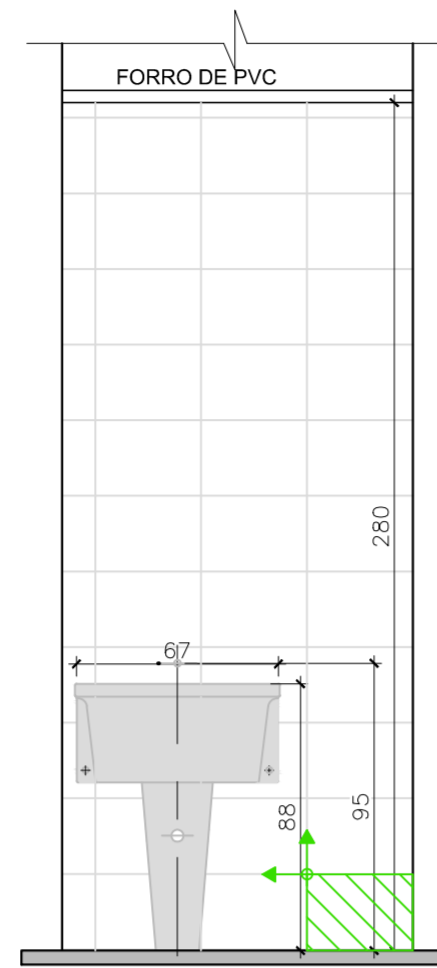
VISTA 02- DML LAVANDERIA "SUJA" ESC.: 1:25
