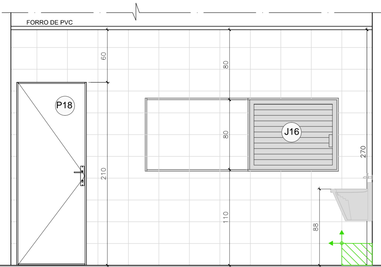
VISTA 04- LAVANDERIA "SUJA" ESC.: 1:25
