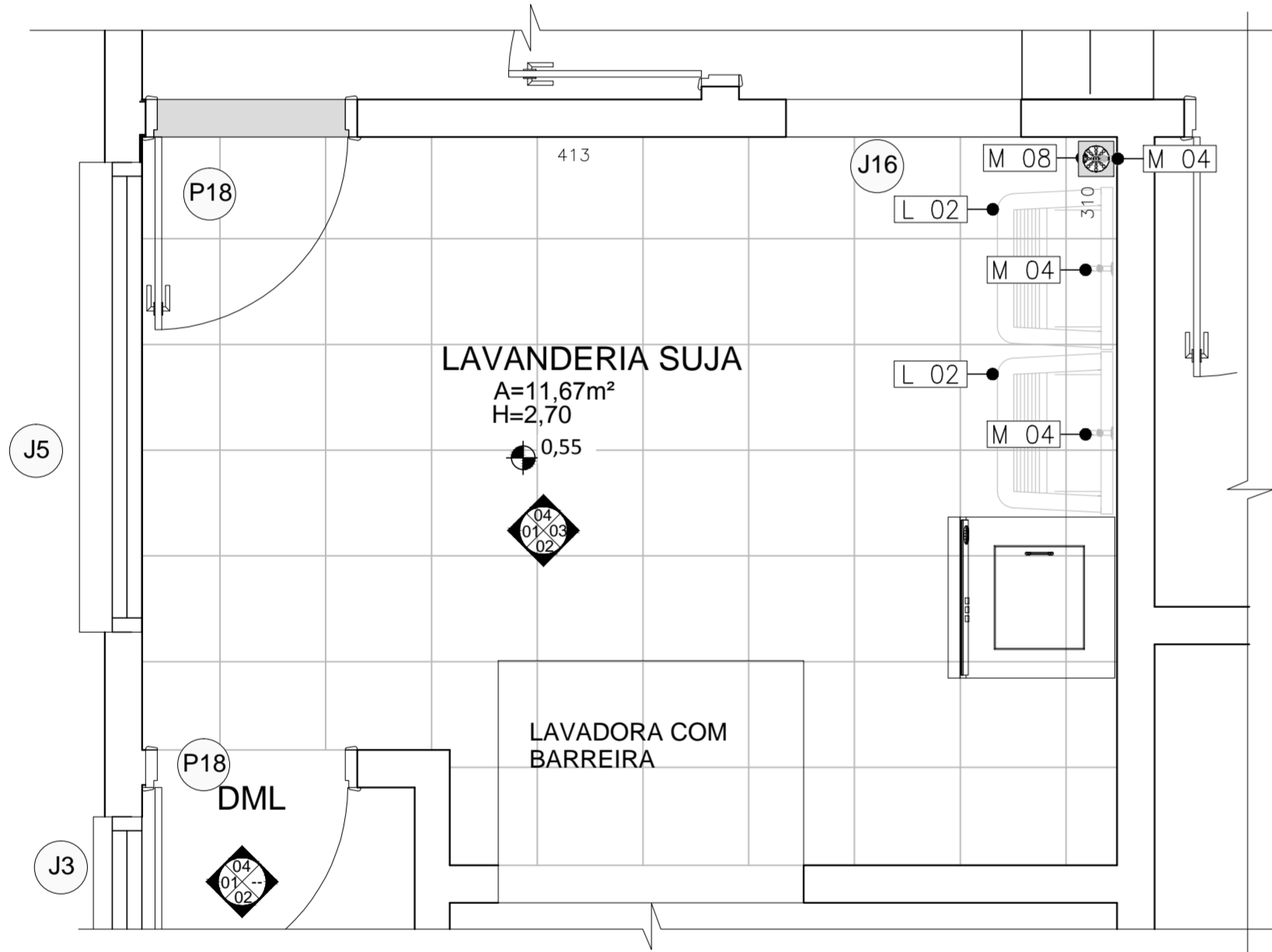
PLANTA BAIXA - LAVANDERIA "SUJA" ESC.: 1:25
