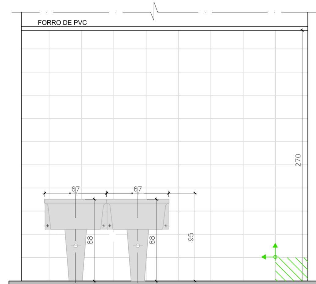
VISTA 03- LAVANDERIA "SUJA" ESC.: 1:25
