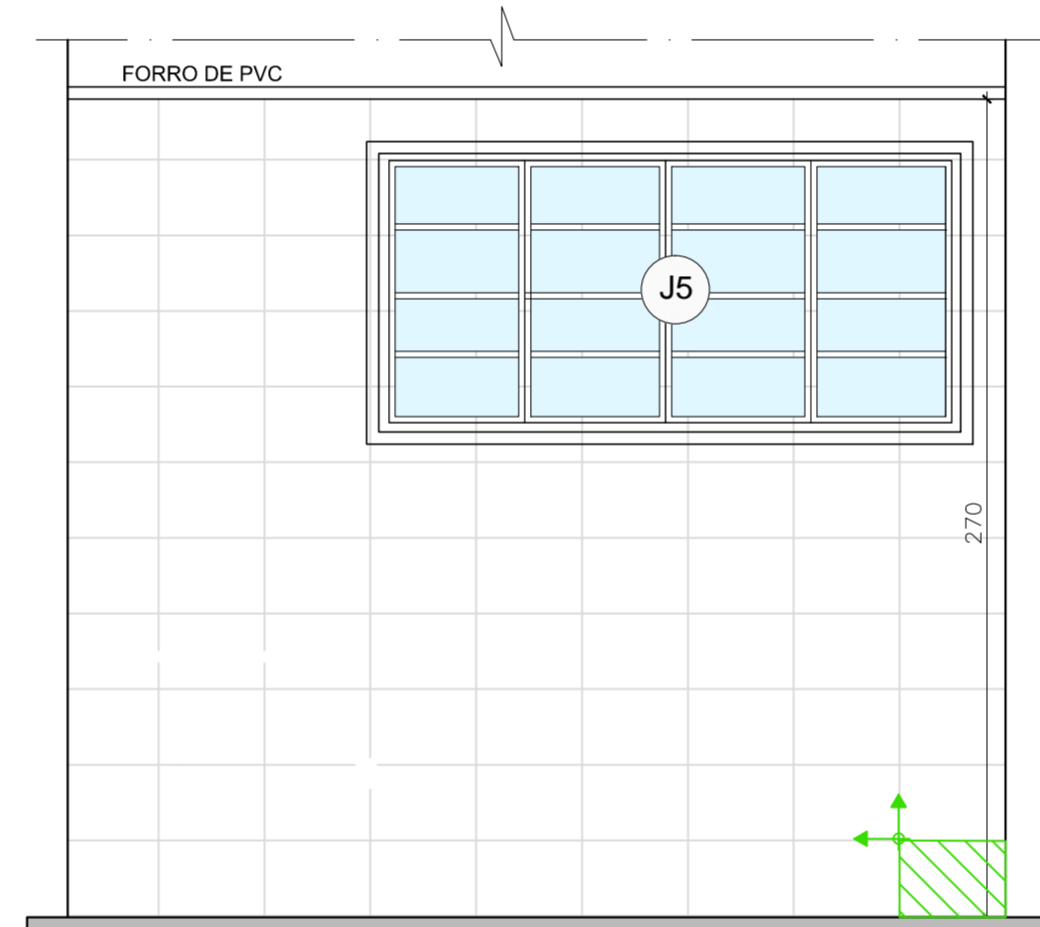
VISTA 01- LAVANDERIA "SUJA" ESC.: 1:25
