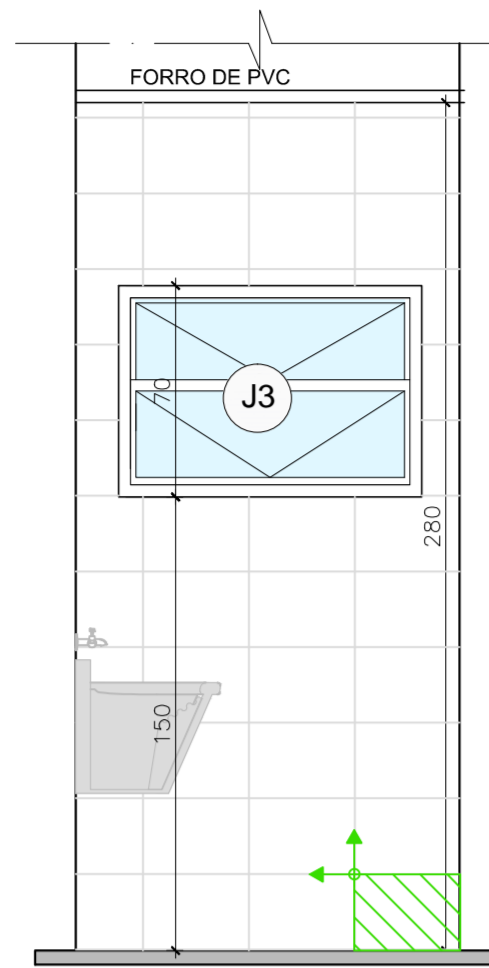
VISTA 01- DML LAVANDERIA "SUJA" ESC.: 1:25
