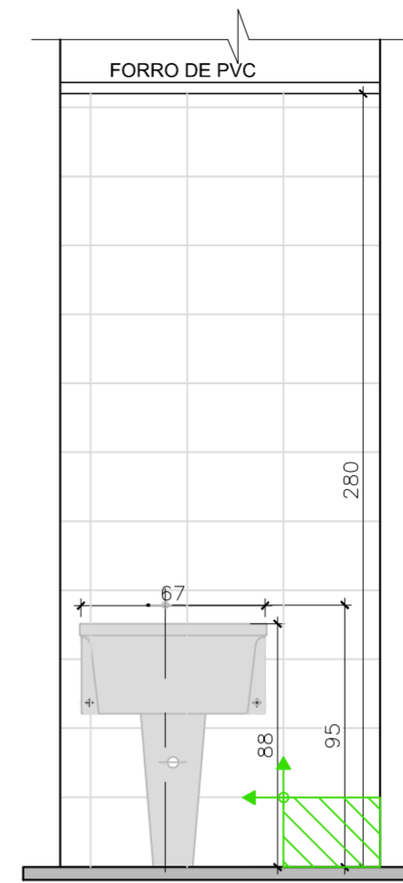
VISTA 04- DML LAVANDERIA "LIMPA" ESC.: 1:25
