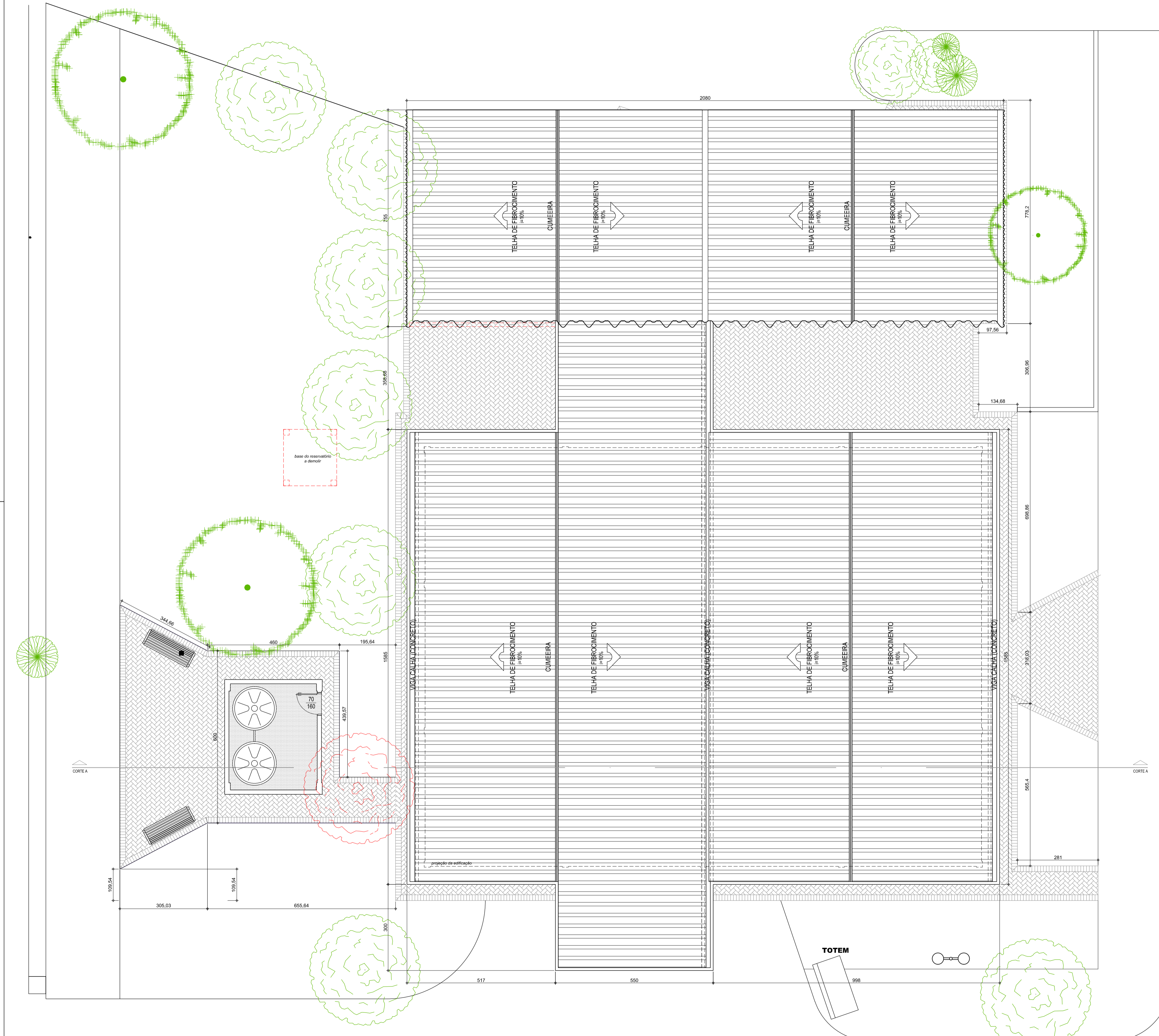
2 PLANTA DE COBERTURA esc. 1/25
