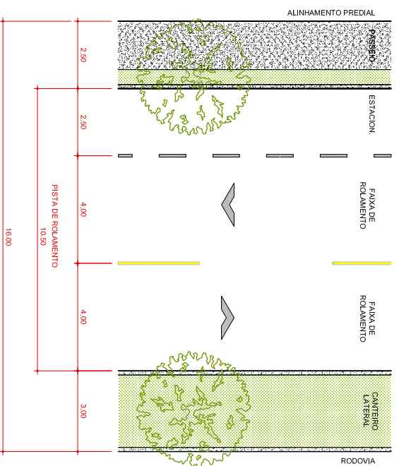
PLANTA VIA MARGINAL DE RODOVIA Escala: 0, 0,50m, 1m, 2m, 3m ESCALA GRAFICA
