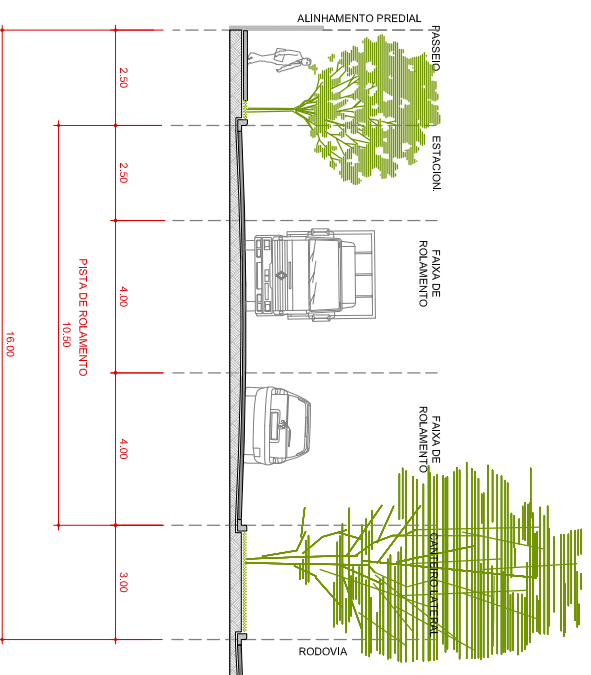
PERFIL VIA MARGINAL DE RODOVIA Escala: 0, 0,50m, 1m, 2m, 3m ESCALA GRAFICA
