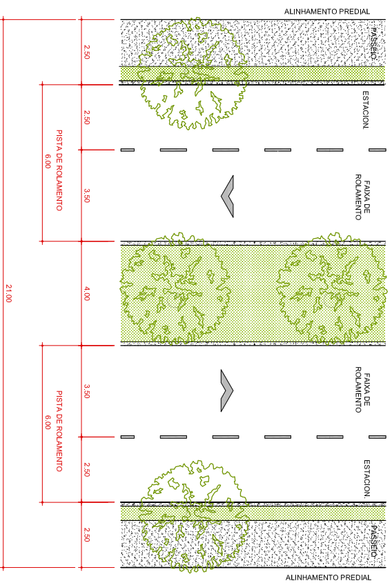
PLANTA VIA ESTRUTURAL ESCALA: 0, 0.5m, 1m, 2m, 3m ESCALA GRAFICA
