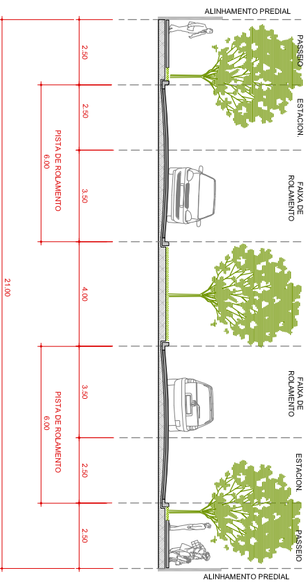
PERFIL VIA ESTRUTURAL ESCALA: 0, 0.5m, 1m, 2m, 3m
