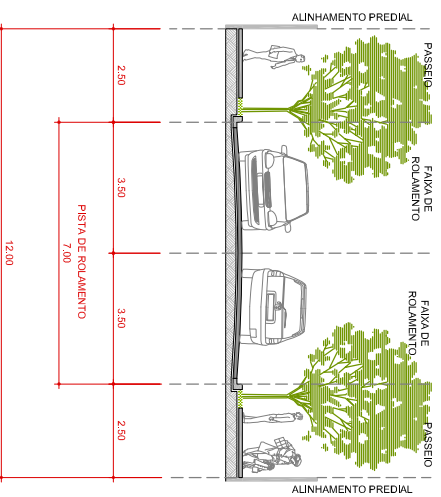
PERFIL VIA DE ESTRUTURAÇÃO MUNICIPAL ESCALA: 0,50m = 1cm ESCALA GRAFICA
