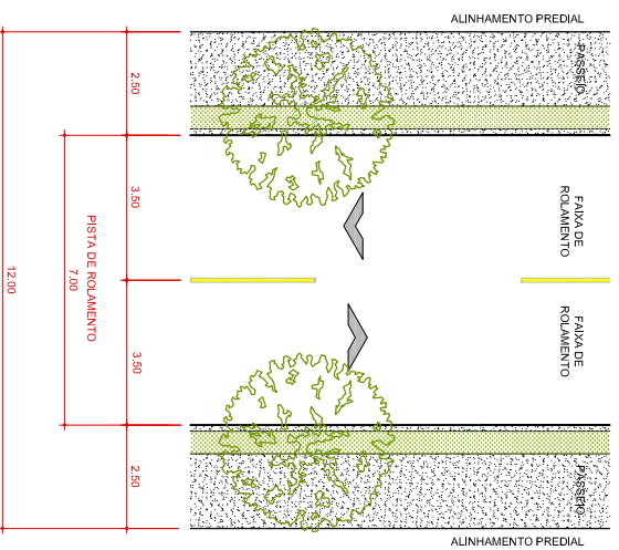
PLANTA VIA DE ESTRUTURAÇÃO MUNICIPAL ESCALA: 0,50m = 1cm ESCALA GRAFICA
