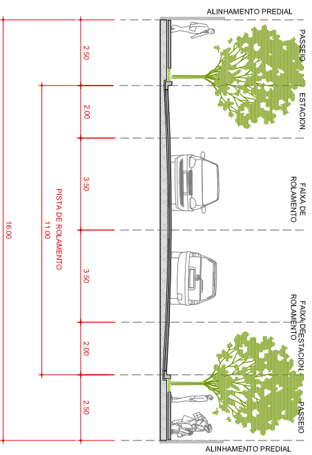
PERFIL VIA COLETORA 0m 2m 4m 6m 8m 10m 12m 14m 16m ESCALA GRAFICA
