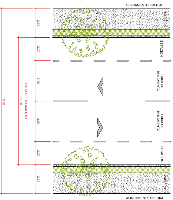
PLANTA VIA COLETORA 0m 2m 4m 6m 8m 10m 12m 14m 16m ESCALA GRAFICA
